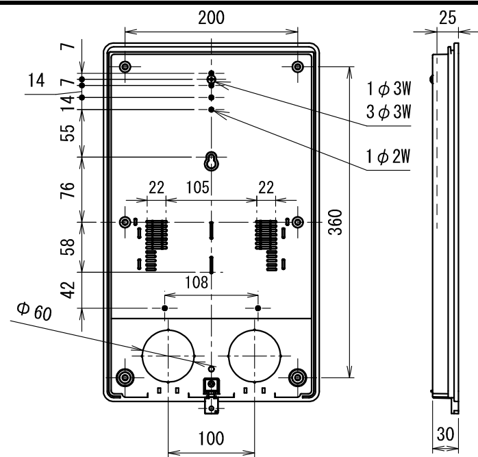
基台(取付板)
